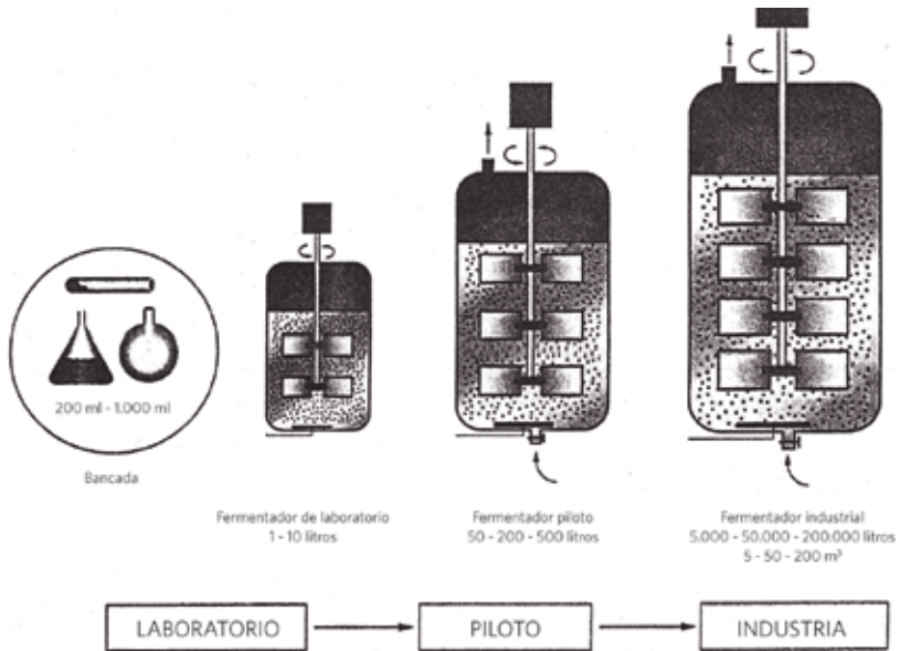
Figura 3.2 El cambio de escala entre el proceso del laboratorio y el proceso industrial origina varios problemas de índole tecnológica (Extraído de Muñoz de Malajovich pág. 119).
