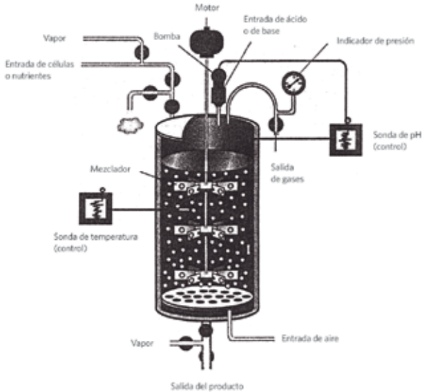
Figura 3.1 Modelo de biorreactor para fermentaciones sumergidas (Extraído de Muñoz de Malajovich, pág. 116).
